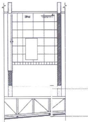
SISTEMA DE EXAUSTÃO - PNE FEMININO E MASCULINO
