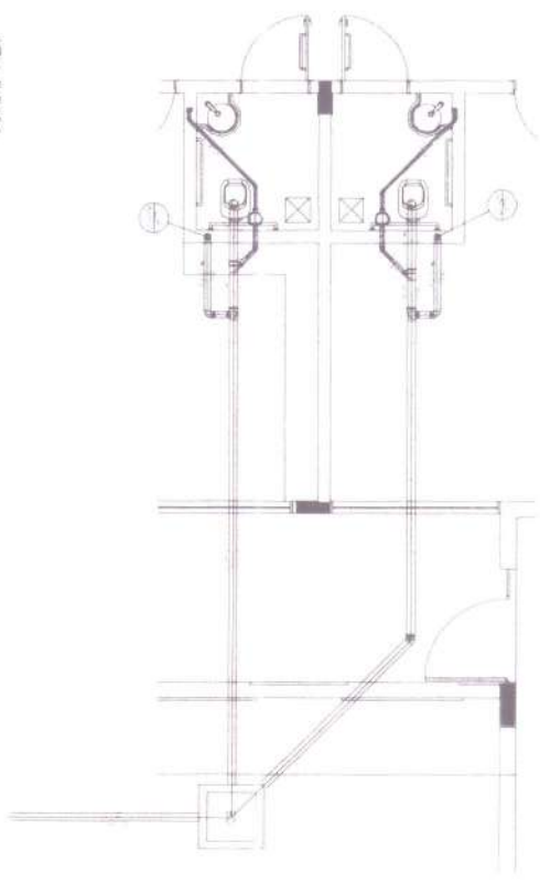
Detalhe S10 escala 1:25
