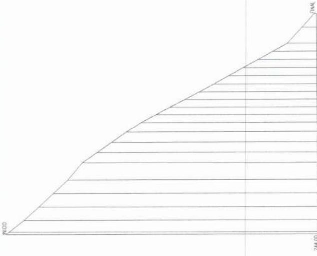
09 PERFIL RUA 01 ESC.: 1/2000
