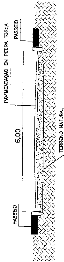
03 PERFIL TRANS esc: 1/75
