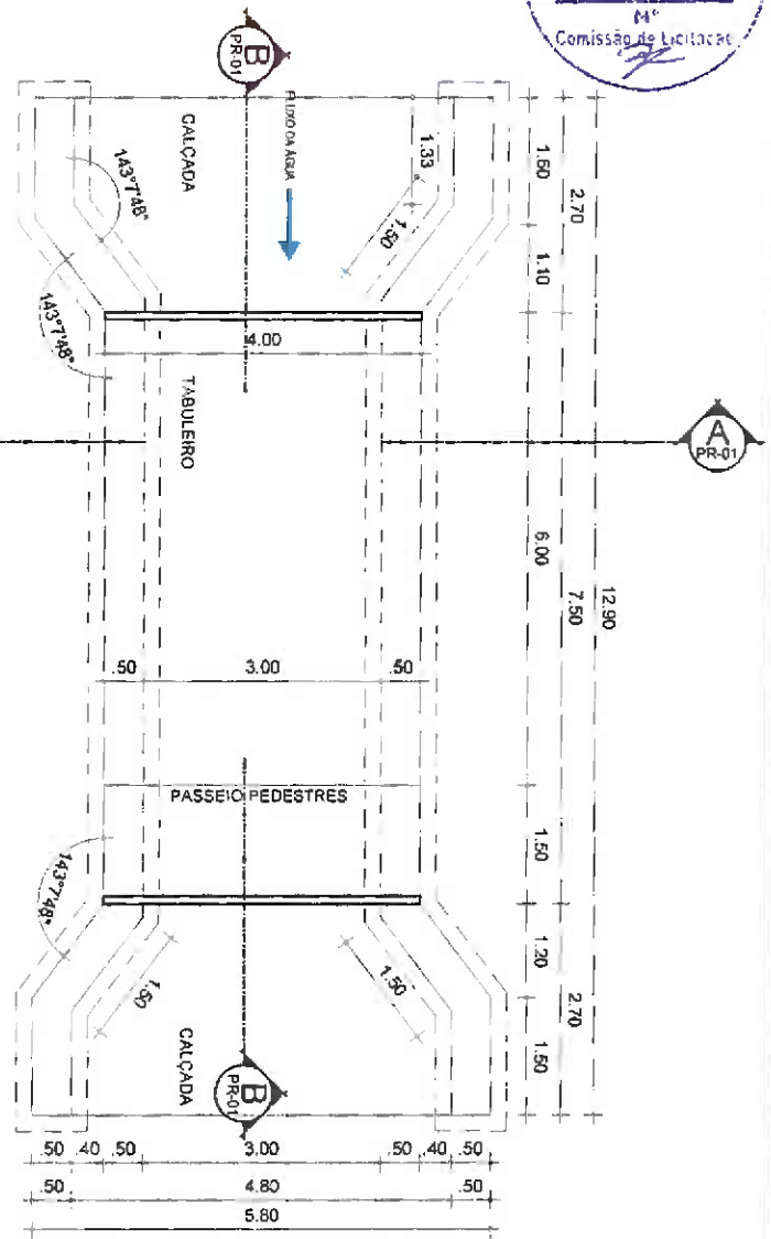
01 PLANTA BAIXA
