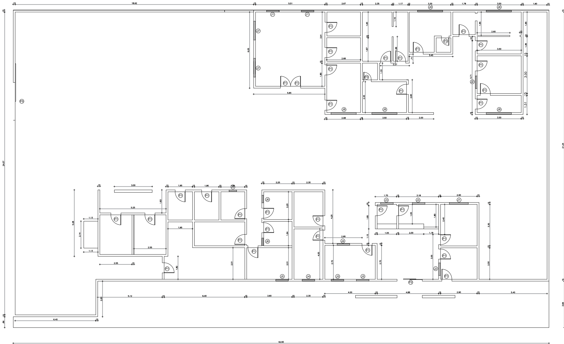
01 PLANTA BAIXA esc: 1/100
