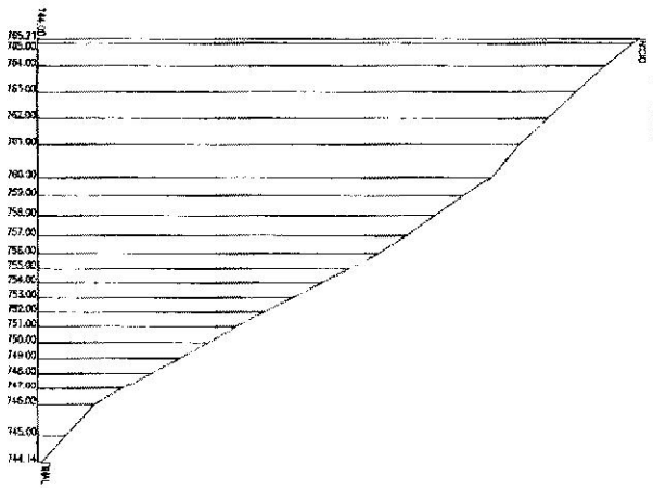
09 PERFIL RUA 01 esc: 1/2000
