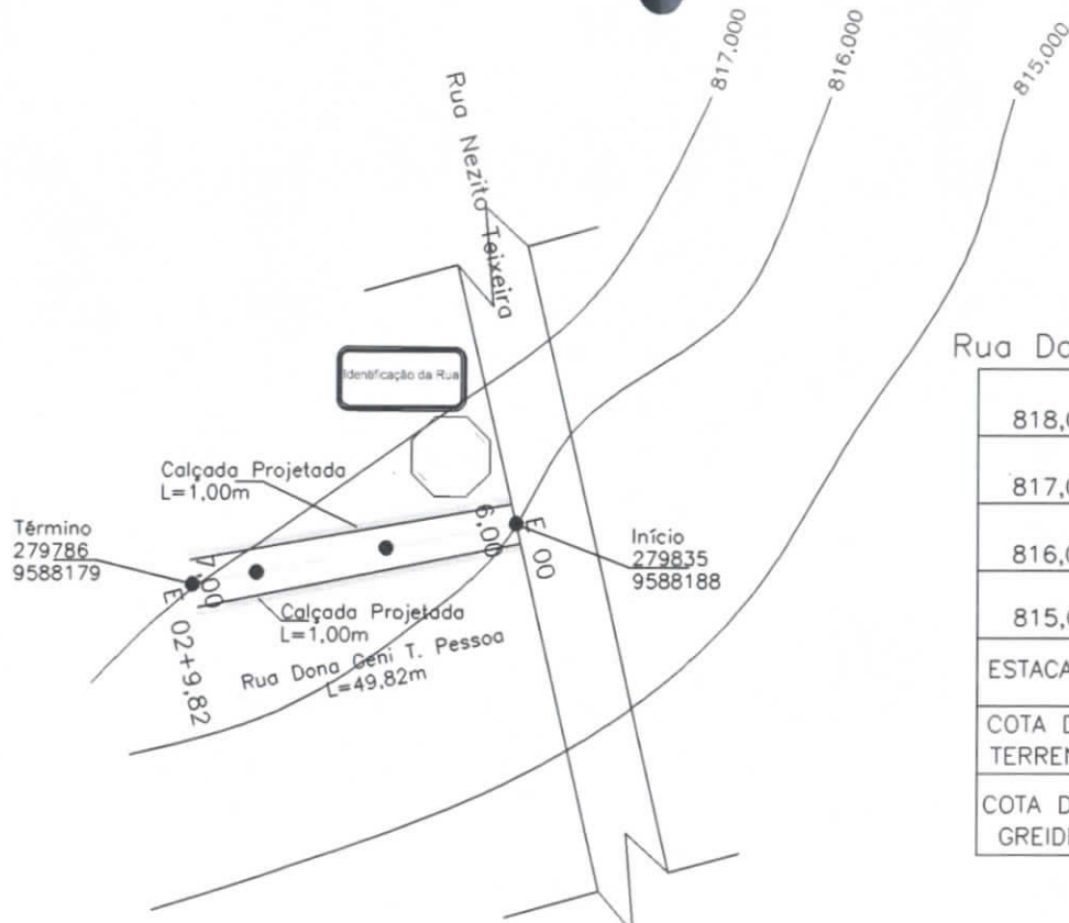
1 PLANTA s/ escala
