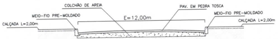
4 PERFIL TRANSVERSAL SEM ESCALA
