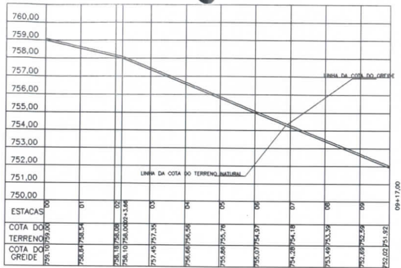
3 PERFIL LONGITUDINAL SEM ESCALA
