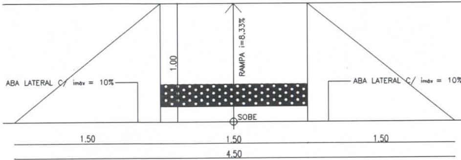
1 DETALHE RAMPA ACESSIBILIDADE s/ escala
