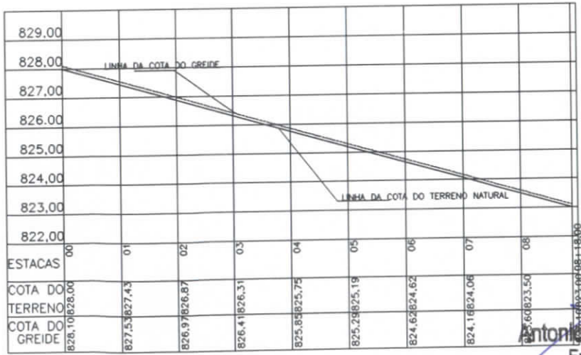
2 PERFIL LONGITUDINAL SEM ESCALA
