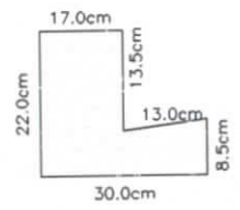
5 DETALHE DO MEIO-FIO SEM ESCALA
