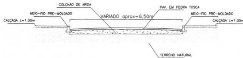
3 PERFIL TRANSVERSAL s/ escala
