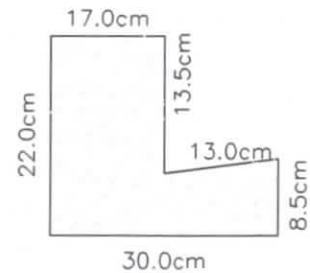
2 PERFIL LONGITUDINAL s/ escala
