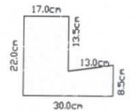
5 DETALHE DO MEIO-FIO SEM ESCALA
